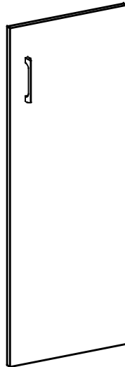
B520(R) 1131x422x18
