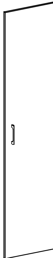
B530 1900x422x18
