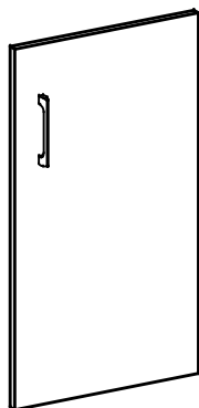
B510(R) 765x422x18
