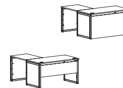
XQPCST 1415/H 1400 x 1500 x 750 XQPCST 1615/H 1600 x 1500 x 750
