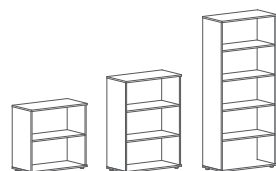
ELCS 85 852 x 430 x 832 EMCS 85 852 x 430 x 1199 EHCS 85 852 x 430 x 1967
