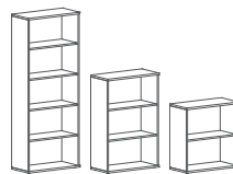
СТ-1 770 x 365 x 1975 СТ-2 770 x 365 x 1200 СТ-3 770 x 365 x 823
