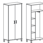
B 701.2/ B 701.2(RZ) 900 x 450 x 2054
