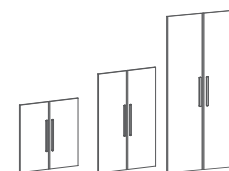
ULD 38-2 764 x 16 x 765 UMD 38-2 764 x 16 x 1132 UHD 38-2 764 x 16 x 1900
