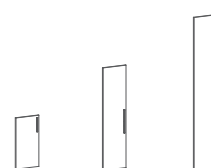
VRD 40-1 394 × 18 × 734 VRMD 40-1 394 × 18 × 1470 VRHD 40-1 394 × 18 × 2206
