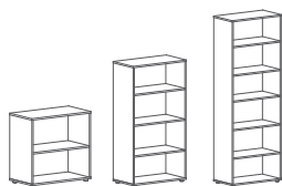
VLCS 80 800 × 430 × 781 VMCS 80 800 × 430 × 1517 VHCS 80 800 × 430 × 2253
