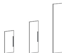
ULD 38-1 381 x 16 x 765 UMD 38-1 381 x 16 x 1132 UHD 38-1 381 x 16 x 1900
