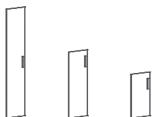
FHD 40-1(L/R) 396 x 18 x 1932 FMD 40-1(L/R) 396 x 18 x 1164 FLD 40-1(L/R) 396 x 18 x 766
