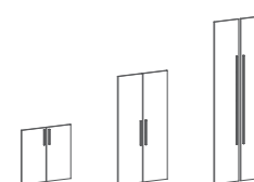
VRD 40-2 790 × 18 × 734 VRMD 40-2 790 × 18 × 1470 VRHD 40-2 790 × 18 × 2206
