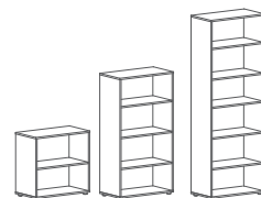
VLCS 80 800 x 430 x 781 VMCS 80 800 x 430 x 1517 VHCS 80 800 x 430 x 2253
