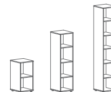
VLCS 40 400 x 430 x 781 VMCS 40 400 x 430 x 1517 VHCS 40 400 x 430 x 2253
